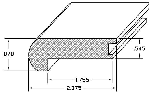
DWG #707 STAIRNOSE
