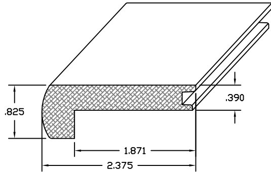
DWG # 700 STAIRNOSE
